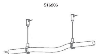
Suspension kit, 2 pcs, adjustable height up to 1,2 m // Aufhängeset, 2 Stück, höhenverstellbar bis 1,2 m
